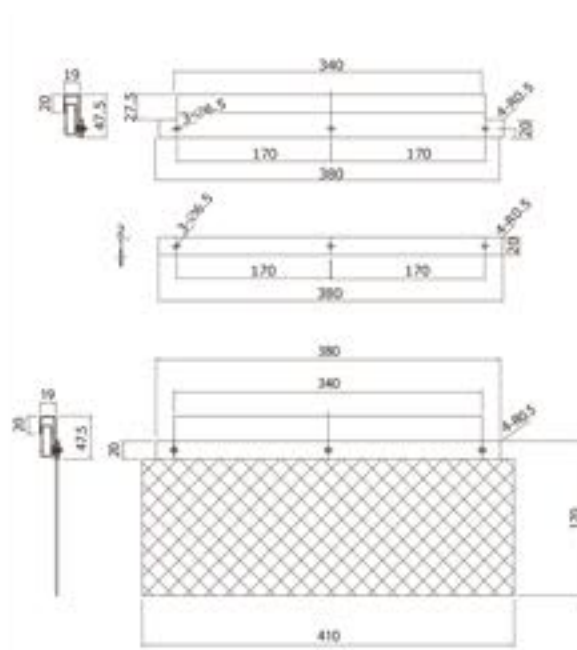
MXGに取り付ける場合
