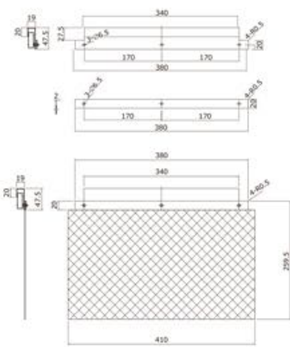
AXG・XXGに取り付ける場合
